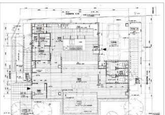
配置図兼 1 階平面詳細図
