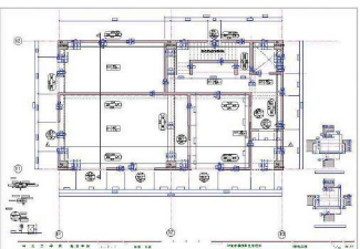
鉄筋コンクリート造躯体図
