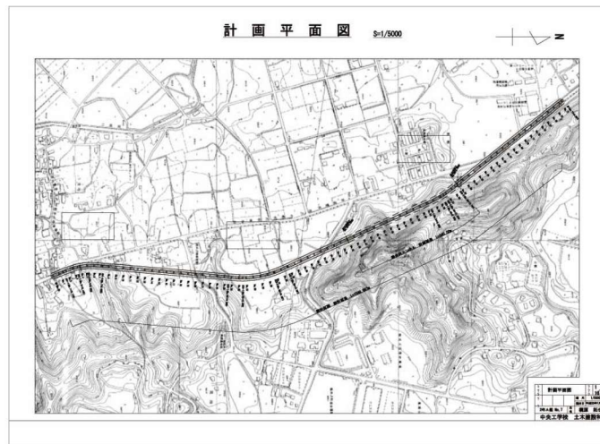
道路平面図
