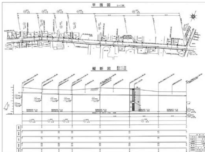
下水道平面図・縦断面図
