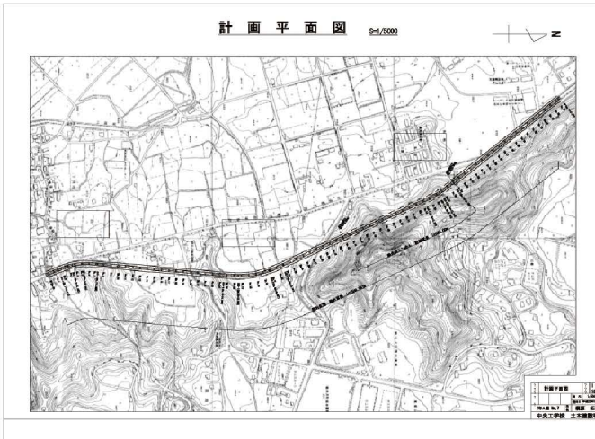
道路設計図（平面）
