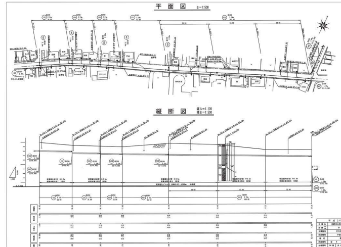
下水道平面図・断面図
